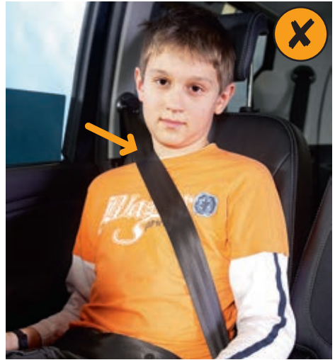
FALSCH: Kind ist zu klein für die Sicherung mit 3-Punkt-Gurt. Der deutliche Gurtkontakt am Hals kann bei einem Unfall zu schweren Verletzungen führen.
